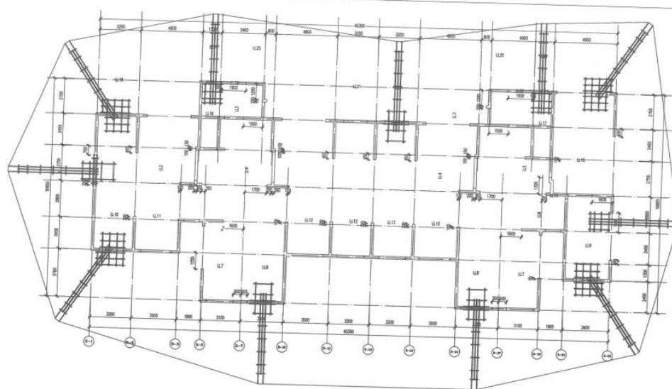
5#楼防护网平面布置图
