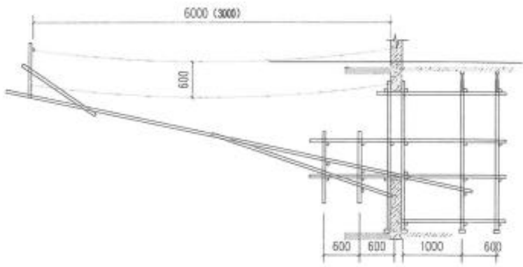
剖面图二
