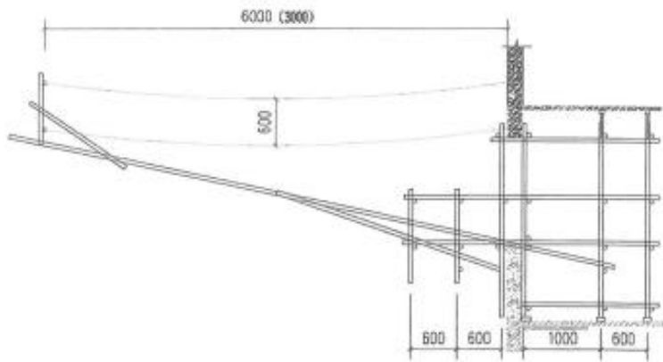
剖面图一
