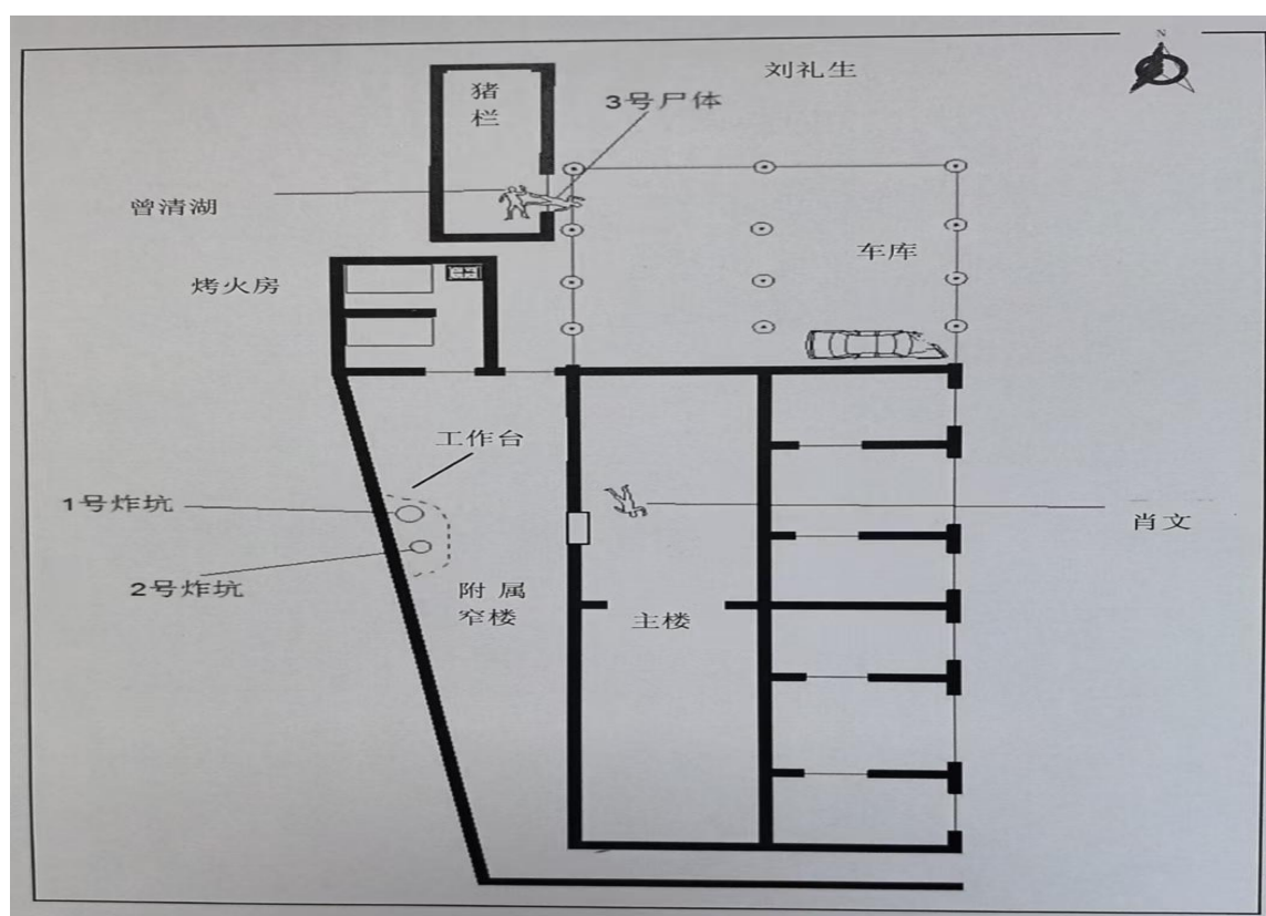
图 3 事故现场平面示意图
