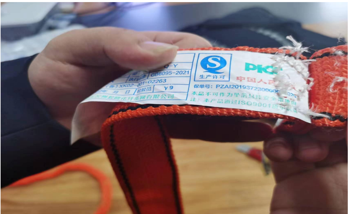
图六、何**所佩戴安全带同款产品（安全带总长 3 米）
