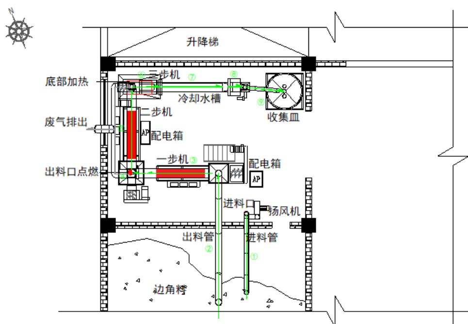
图 5 废塑料再生车间平面图
