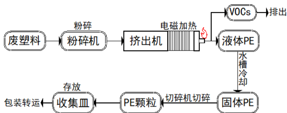
图 6 废塑料再生车间工艺流
