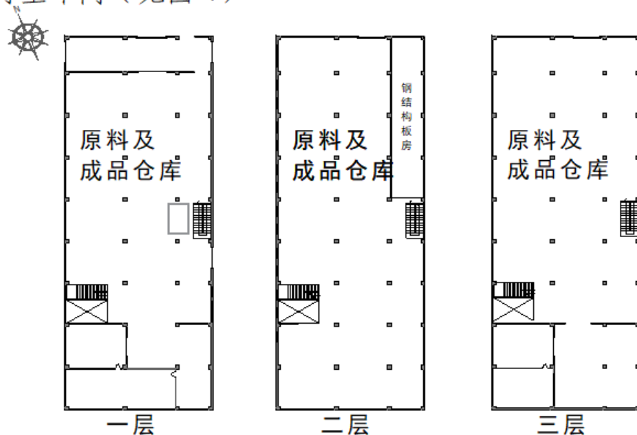
图 4 原料及成品库楼层平面图
