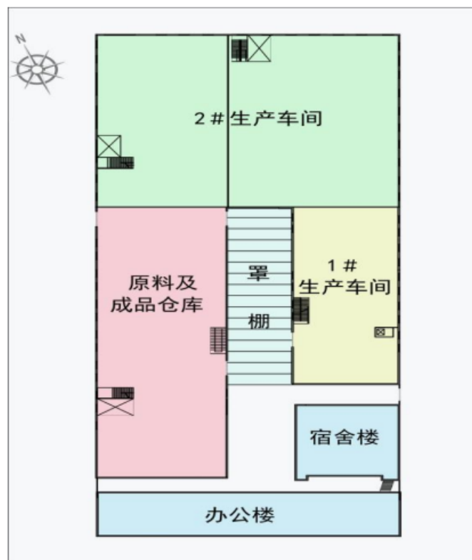
图2 锦中元公司总平面图
