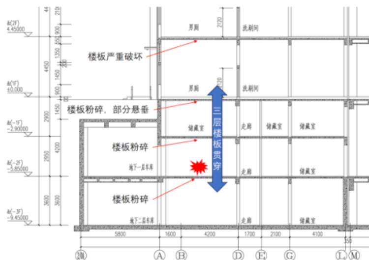
图 1 1 号楼爆炸位置结构剖面图
