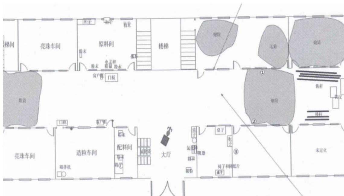
图 3、 爆炸现场平面图
